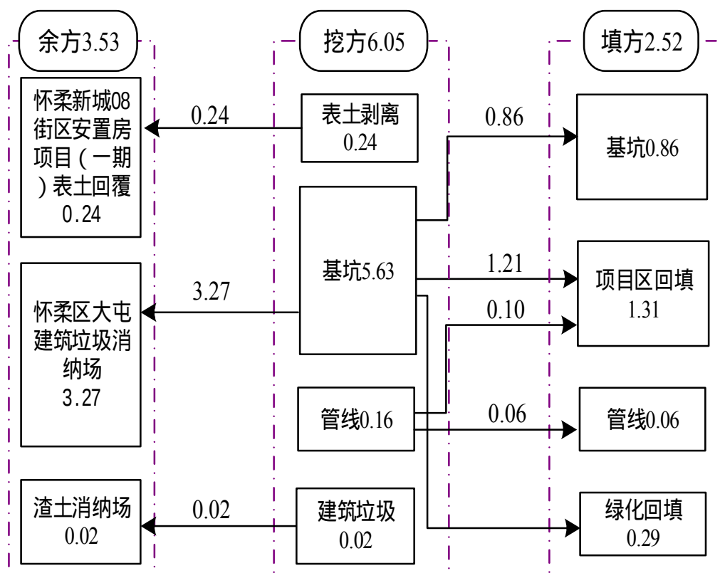
图 2-2 土石方平衡及流向框图
